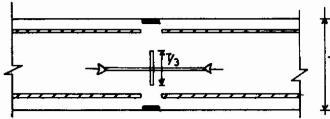
تصویر ۶-۷: اجزاء درز انقباض قائم با آب‌بندکننده صلیبی
